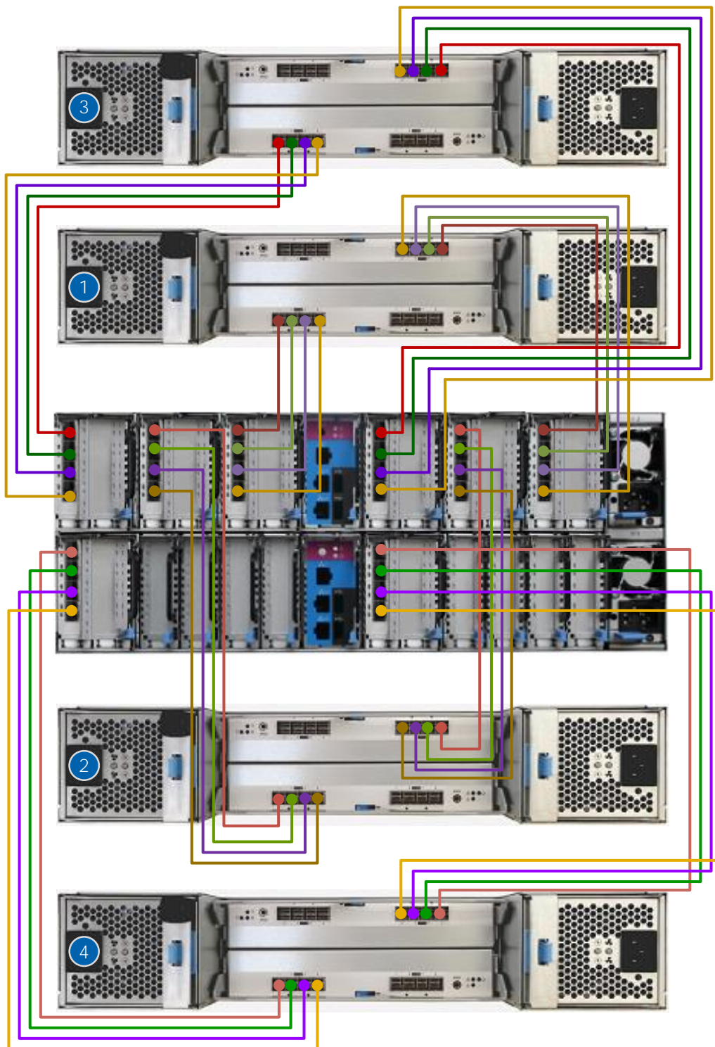
图 5-6 连接 4 台 JBOF 扩展柜（无 ACC）
