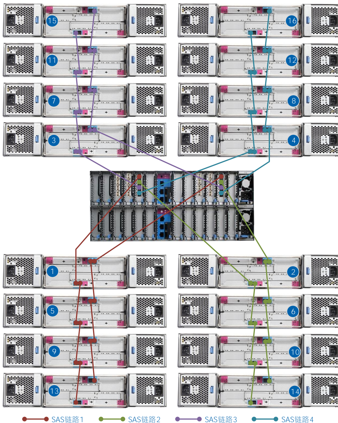
图 5-5 连接 16 台 JBOD 扩展柜（每控 1 张 4 口 SAS 卡）
