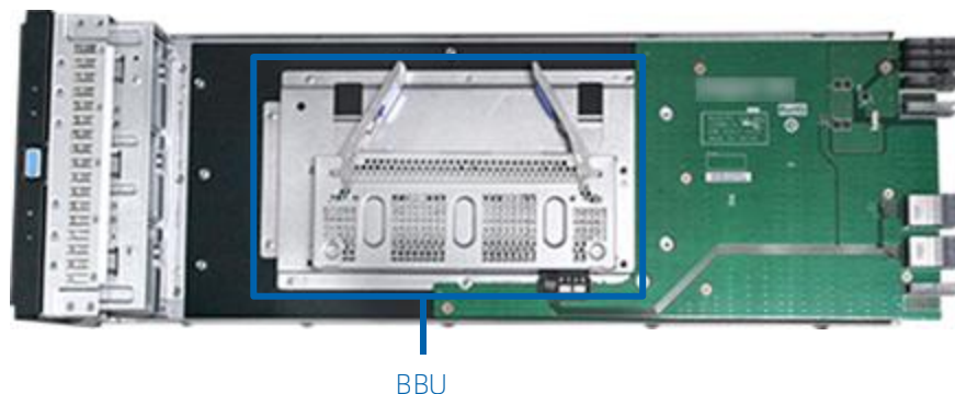
图 2-11 BBU 模块
