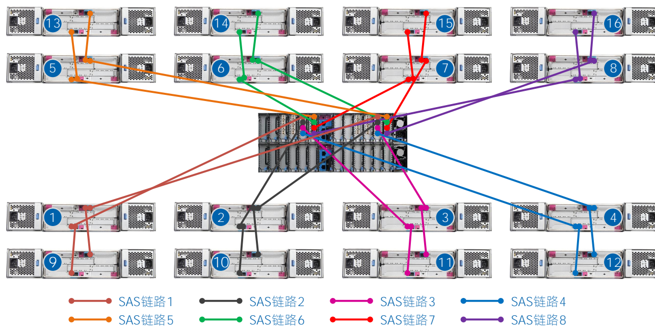
图 5-4 连接 16 台 JBOD 扩展柜（每控 2 张 4 口 SAS 卡）
