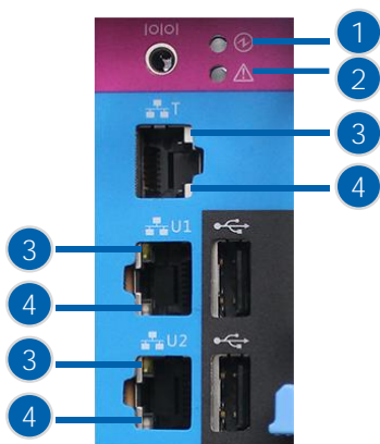
图 4-2 CMC 指示灯
