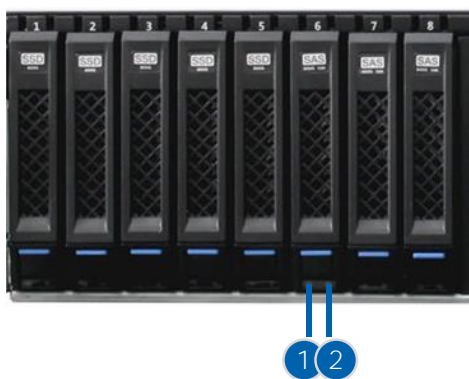
图 4-10 JBOF 硬盘指示灯
