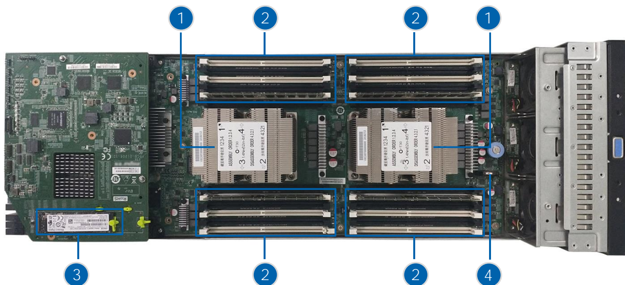
图 2-3 控制器内部结构图
