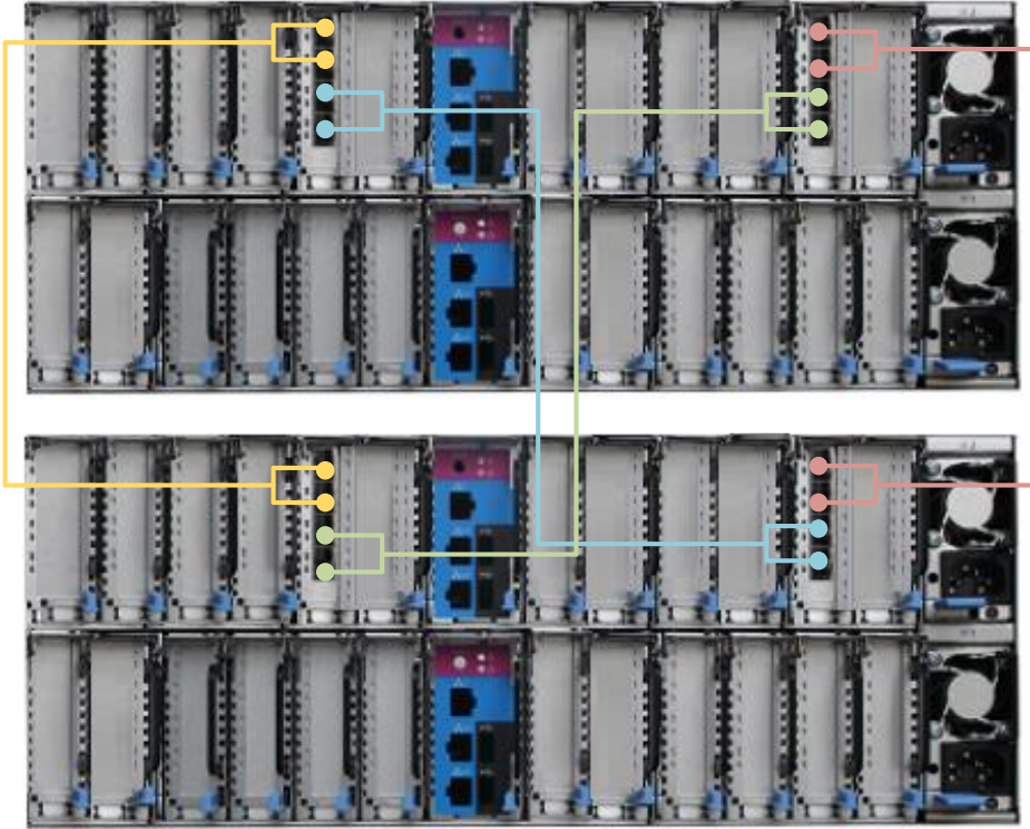
图 5-2 NTB 卡四控连接（双端口线缆方式）
