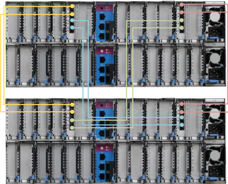
图 5-3 NTB 卡四控连接（单端口线缆方式）
